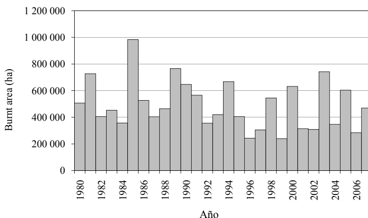
Figura 4. Zonas quemadas en la región mediterránea de la UE.
