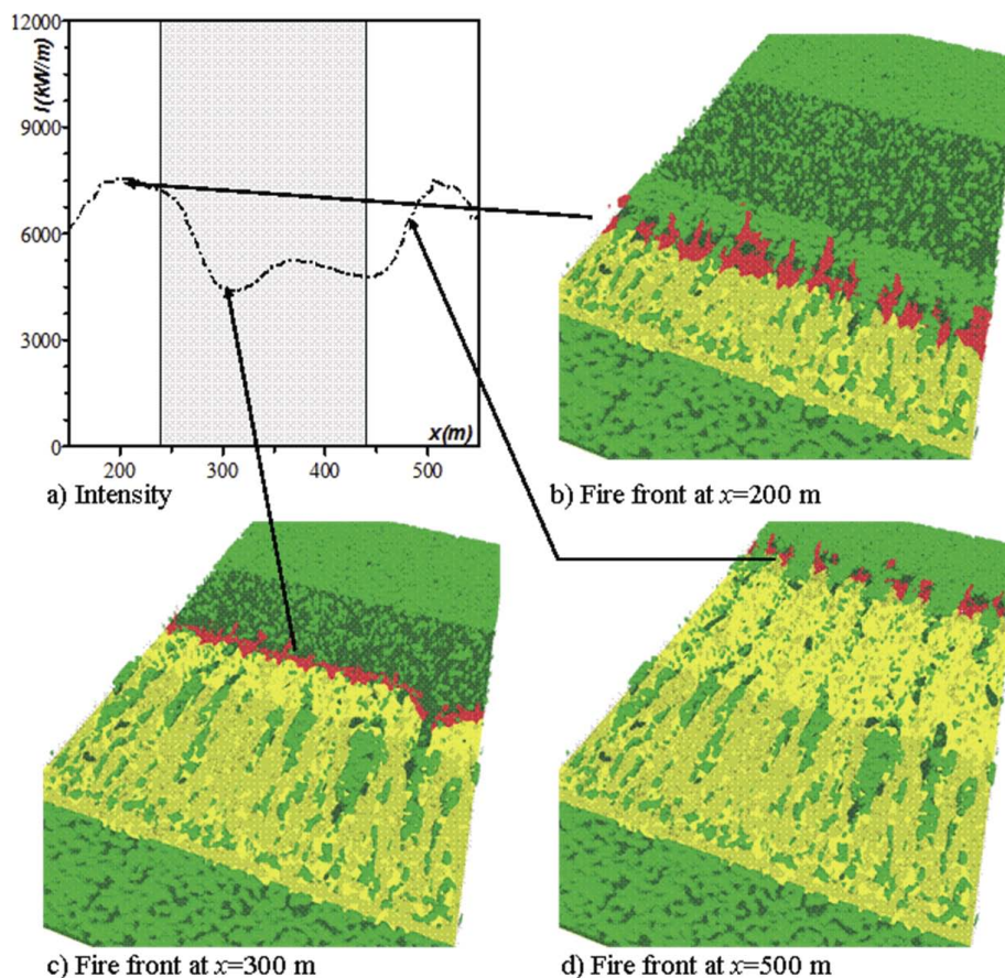
Figura 10. Simulación numérica de la propagación de un fuego sobre un cortafuego en un pinar de P. halepensis , utilizando el modelo acoplado llamado FIRETEC (INRA - LANL trabajo conjunto, Pimont et al. 2008). La fracción de superficie cubierta por árboles en los cortafuegos asciende a un 25%. El fuego se propaga por el eje de las x y el cortafuegos se extiende desde x=240 m hasta x=440 m. Las isotermas computerizadas proporcionan los contornos de las llamas en rojo. El color verde representa la copa de los árboles y el amarillo los combustibles de superficie (arbustos, pasto) (isocontornos de la densidad de biomasa computerizada).
