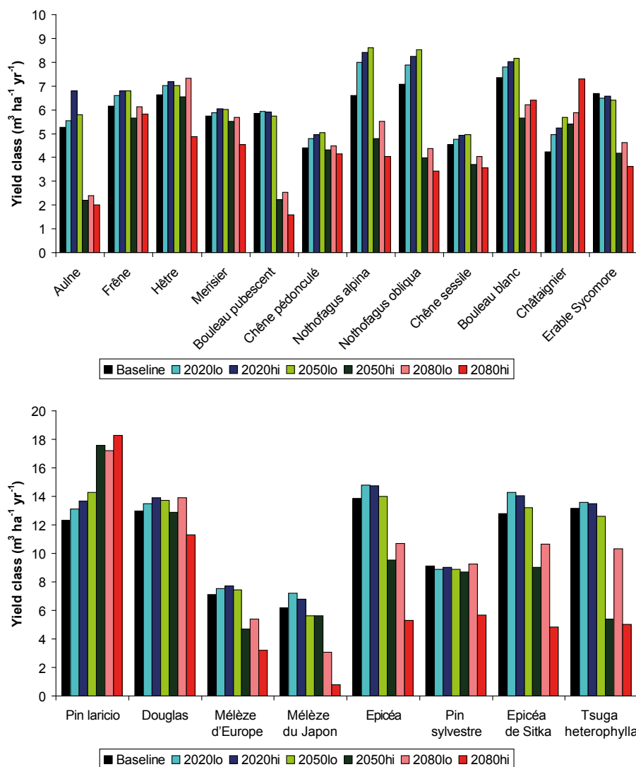
Figure 9. Evolution des rendements de feuillus (en haut) et résineux (en bas) selon différents scénarios d'émission au Royaume Uni (lo : émissions faibles ; hi : émissions élevées). Source : Gardiner, 2011.
