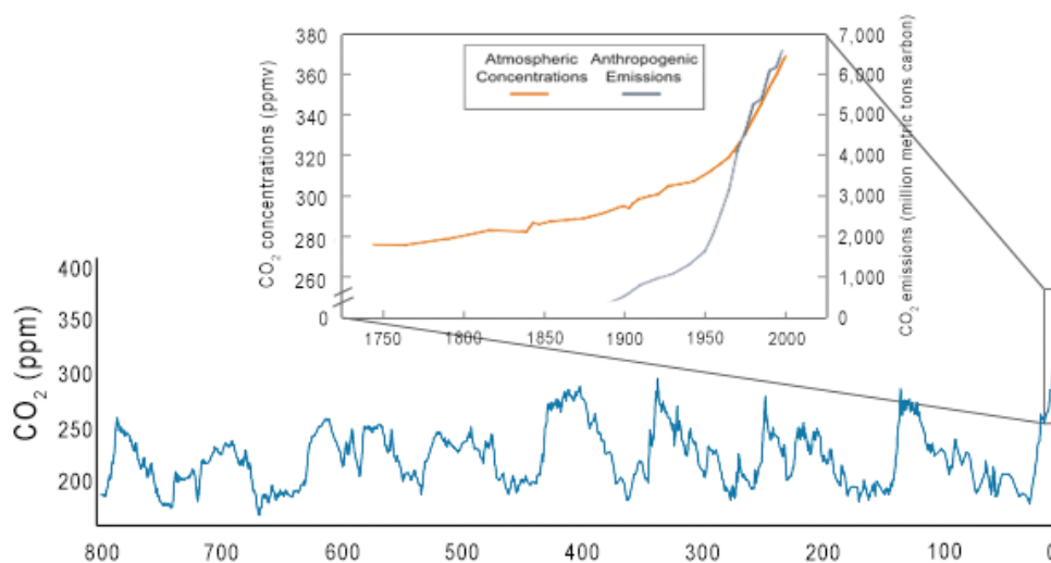
Figure 2 : Evolution des concentrations de \text{CO}_2 depuis 800 000 ans et émissions anthropiques de \text{CO}_2 depuis 150 ans. D'après Oak Ridge National Library, Carbon Dioxide Information Center et Hansen et al. 2008.
